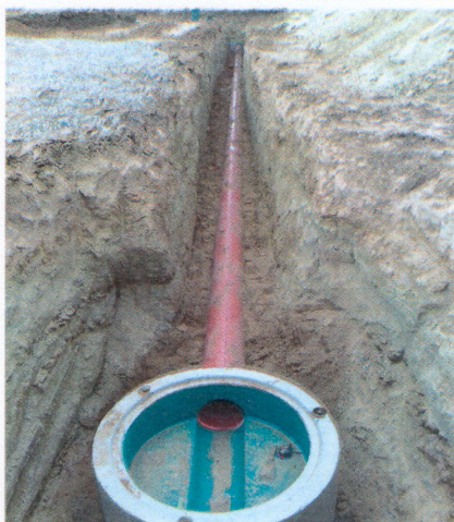
Šachtové dno na kanalizaci
